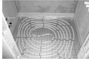
Fußbodenheizung
